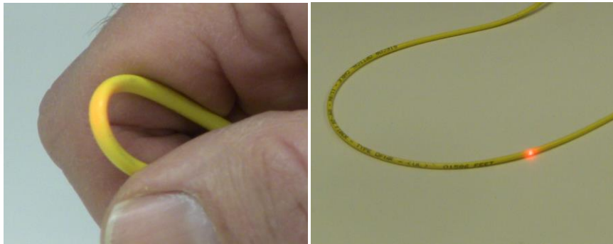
Macrobend
