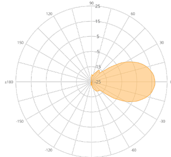
N5-X16 (16 dBi)
