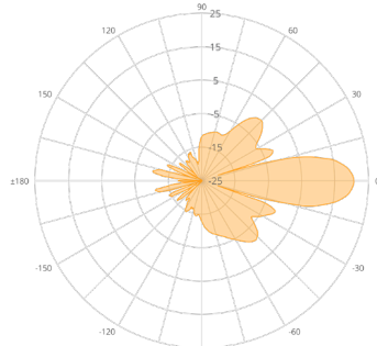
N5-X20 (20 dBi)
