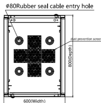
A-A SECTION
