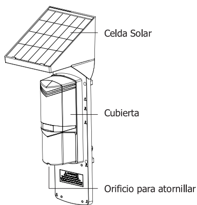
Cubierta frontal
