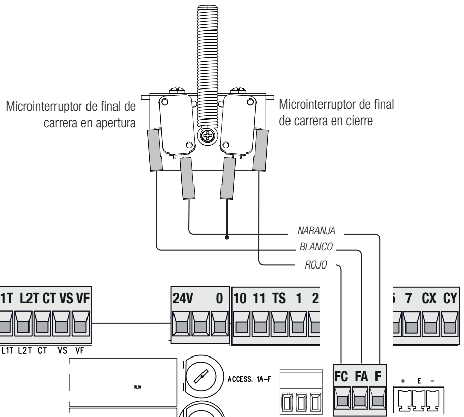
Final de carrera mecánico
