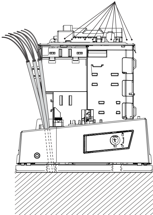
Pasacables del soporte de la tarjeta
