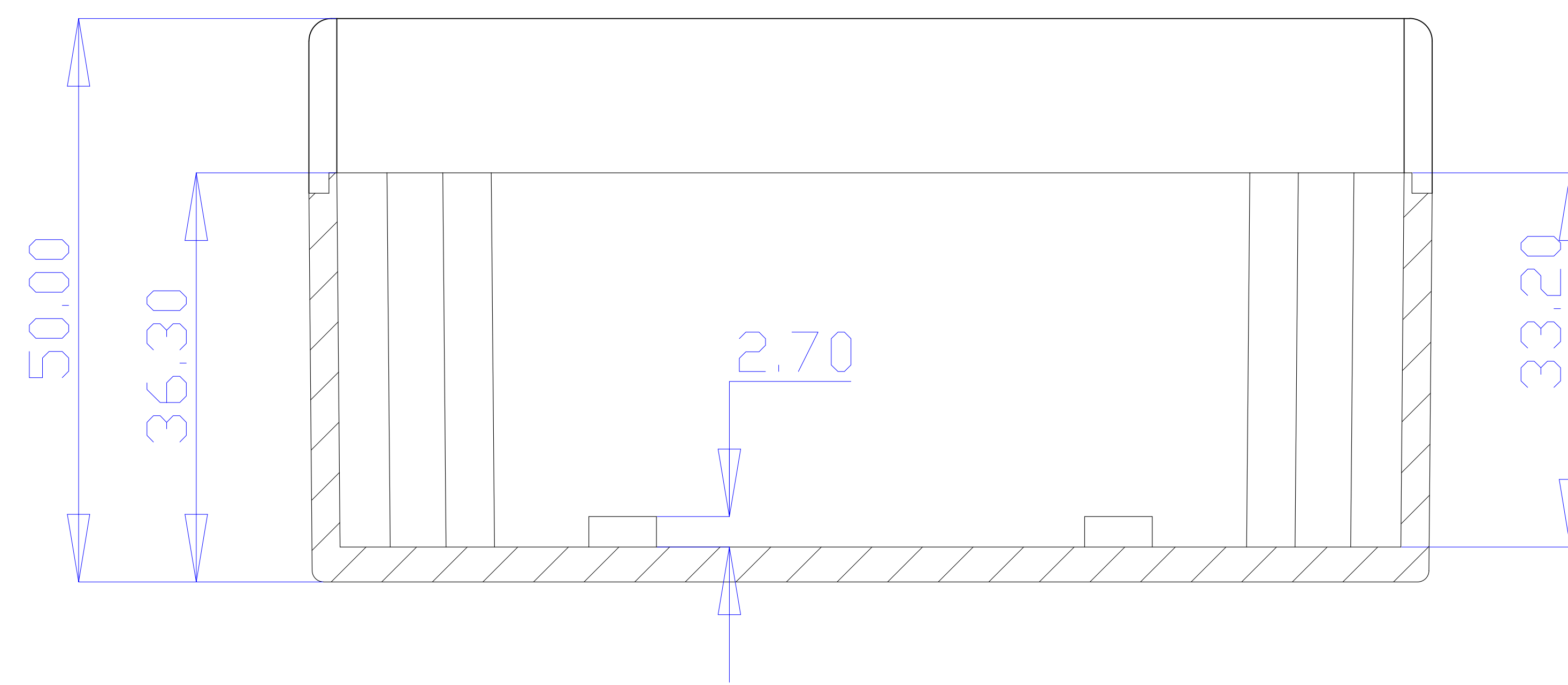
Sección A-A
