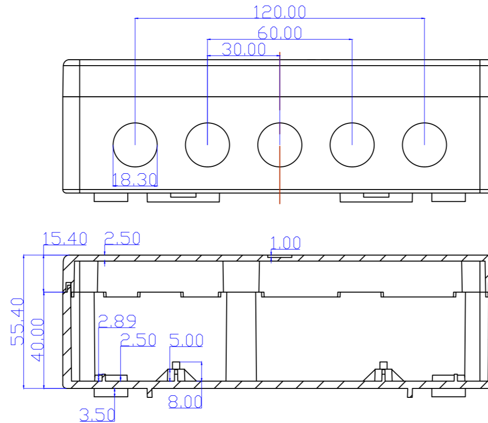
SECCIÓN A-A
