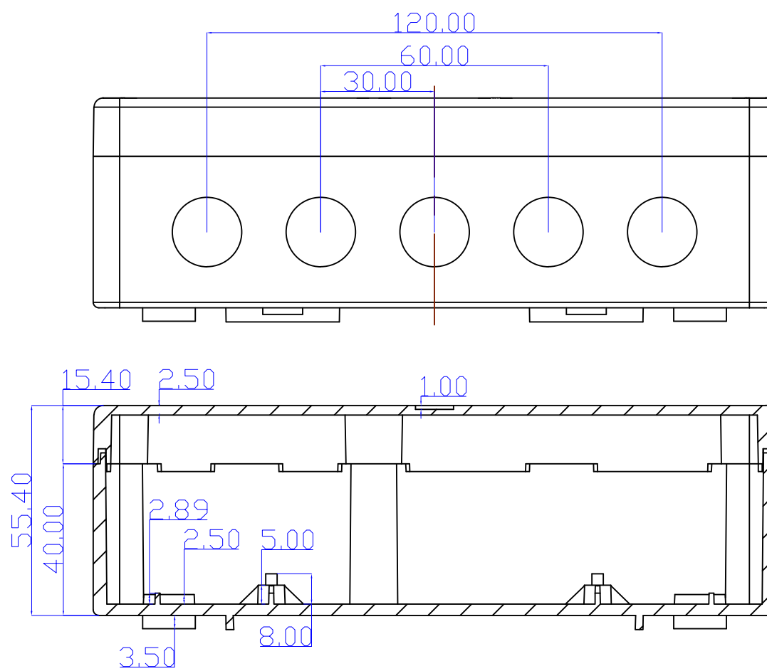
SECCIÓN A-A
