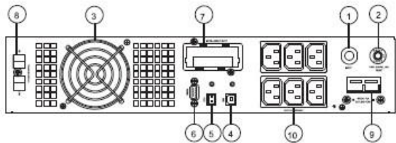
b. 0.9PF 1.5K&2KVA RT Panel Posterior
