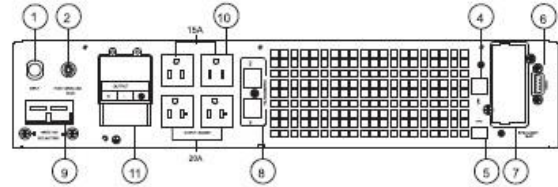
b. 0.9PF 1.5K&2KVA RT Panel Posterior
