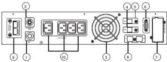
a. 0.9PF 1KVA RT Panel posterior
