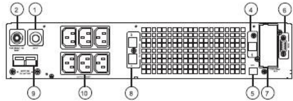
b. 0.9PF 1.5K&2KVA RT Panel posterior
