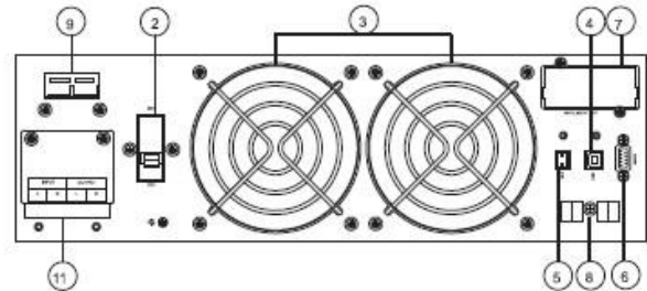
d. 0.9PF 6/10KVA RT Panel posterior
